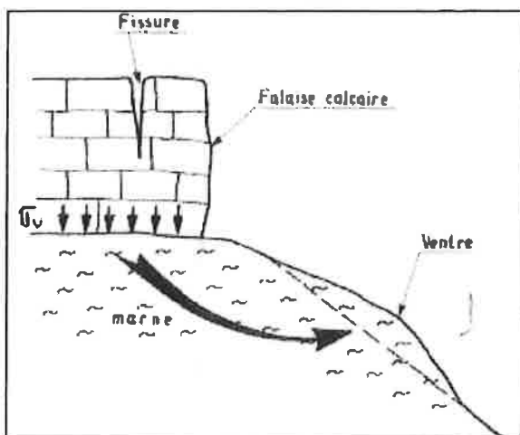
Illustration 4: Fluage d'après Philipponnat & al. (rapport BRGM)
